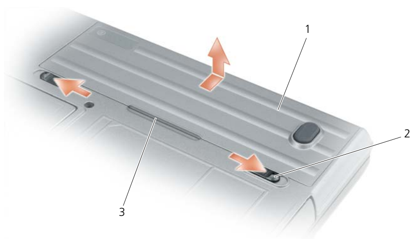
1 バッテリー 2 バッテリーベイリリーススラッチ (2) 3 バッテリータブ
